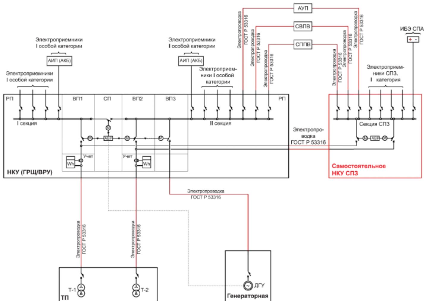
Рисунок А.6 - Структурная схема организации электроснабжения СПЗ при применении самостоятельного НКУ для зданий медицинских организаций, предназначенных для оказания медицинской помощи в стационарных условиях (круглосуточно), класса функциональной пожарной опасности Ф1.1, с ЦОД, со встроенными АКБ, ИБЗ для питания СПА и третьего независимого источника питания (электрогенераторной установки или ИБП) для питания СВПВ, СППВ и АУП
