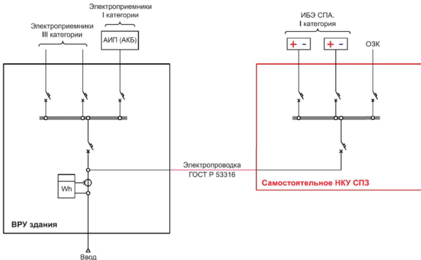
Рисунок А.8 - Структурная схема организации электроснабжения СПЗ на объектах, электроприемники которых отнесены к III категории электроприемников по надежности электроснабжения, где питание СПЗ выполнено с применением АИП (например: ИБЭ с АКБ достаточной емкости), где реализовано управление напряжением сети огнезадерживающим клапаном
