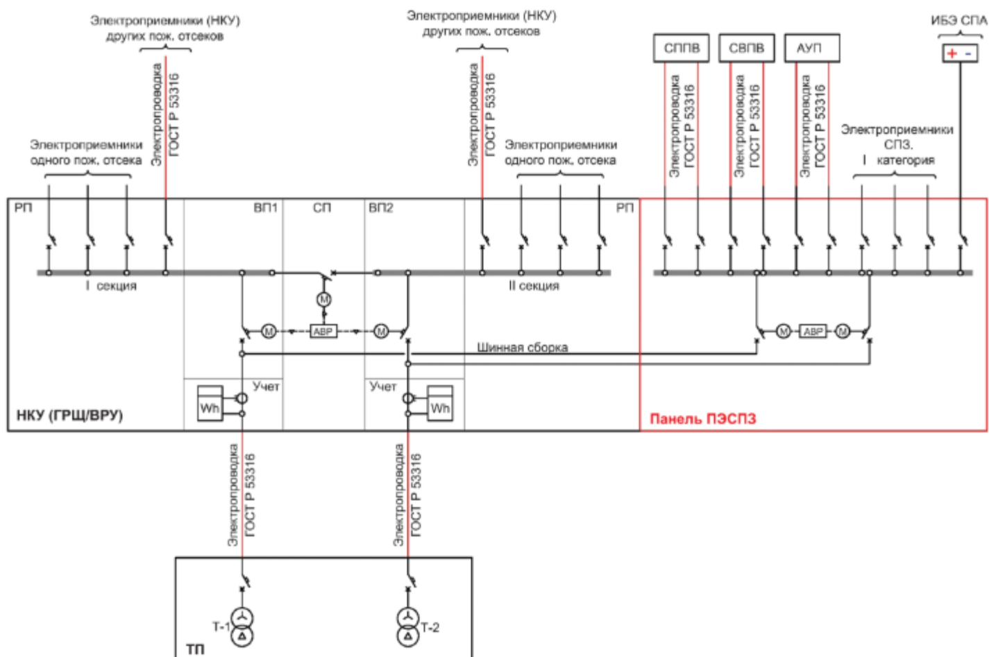
Рисунок А.2 - Структурная схема организации электроснабжения электроприемников I категории надежности и применения самостоятельного НКУ СПЗ
